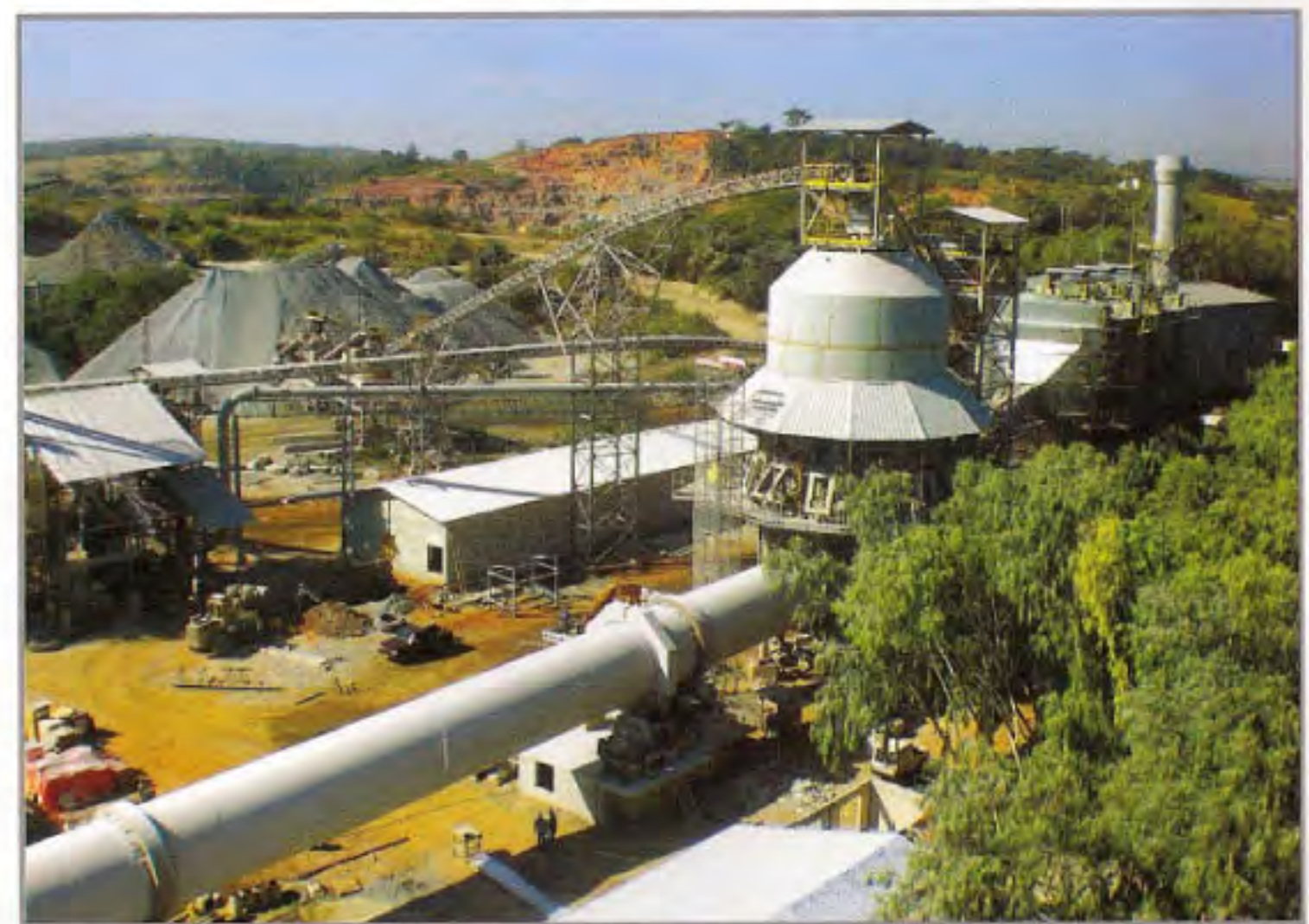
安装中的巴西MG州活性石灰生产线 Brazil MG lime production line under installation
