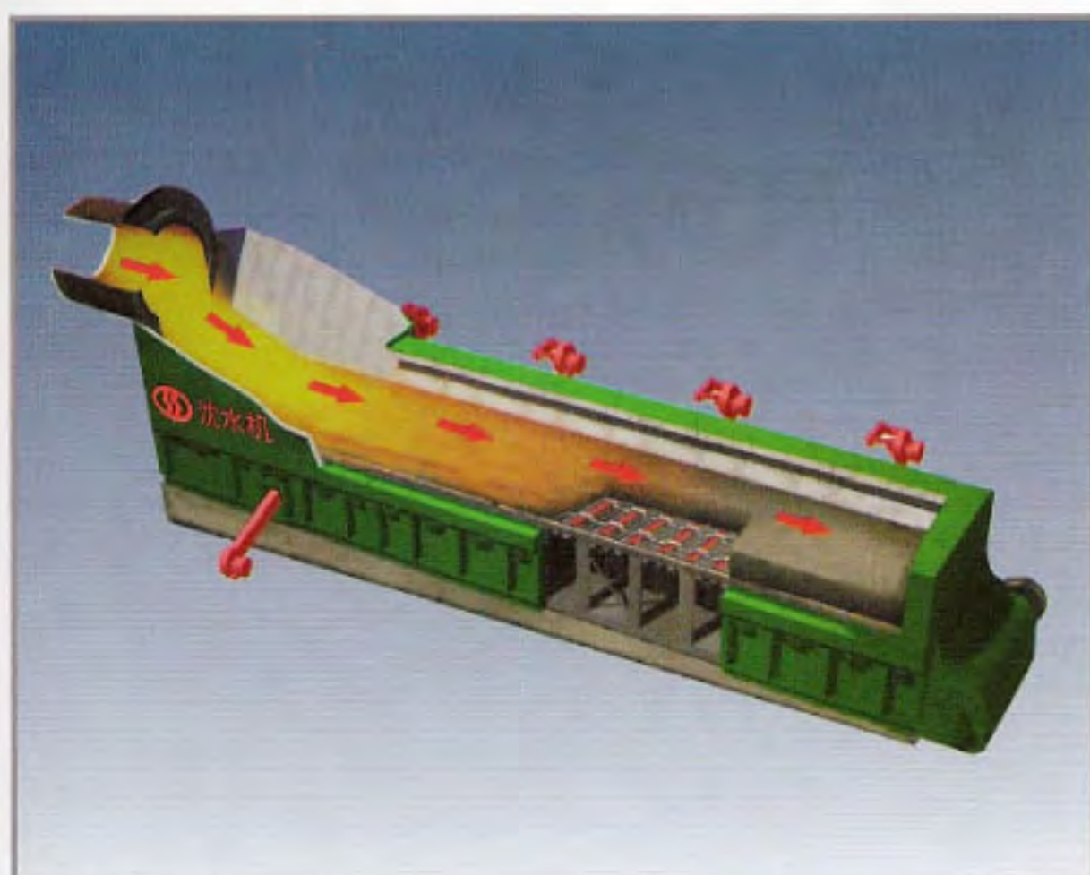
第四代篦冷机 The fourth generation grate cooler
